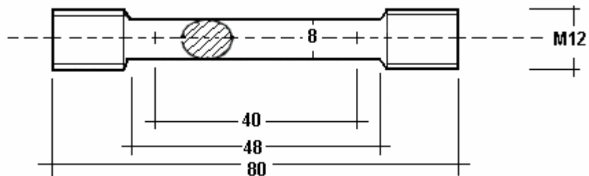
Zkouška tahu
